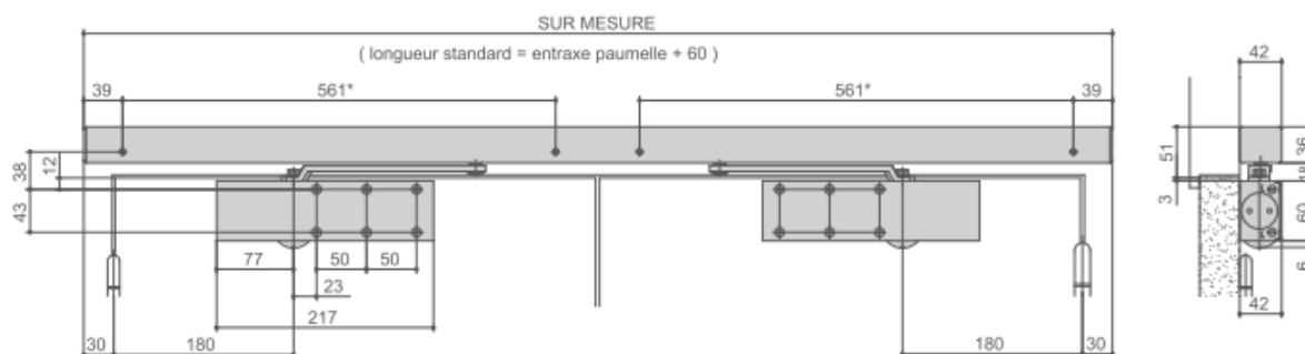
SL 2000 posé coté paumelles avec deux HL105 n°3 * Cotes pouvant évoluer suivant dimension particulière du bandeau.
