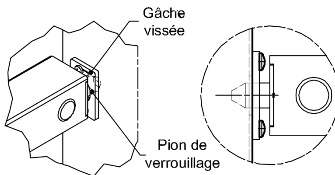
Détail du verrouillage côté montant d'huissierie
